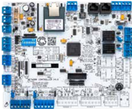
Network 2 Door Controller CSEV02
